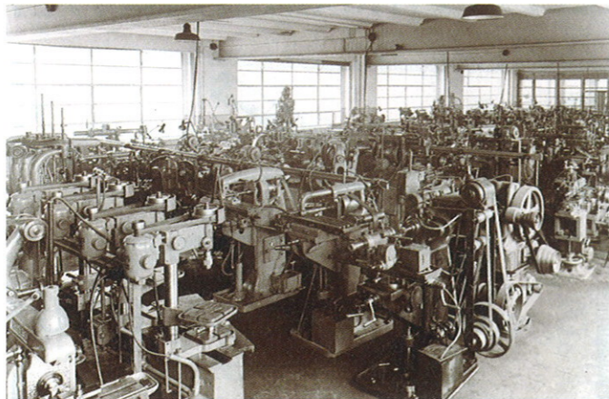
Værkstedshal fra cirka 1930. Bemærk den kompakte opstilling af maskinerne med uafskærmet remtræk. Her var ikke plads til klaustrafobi!
